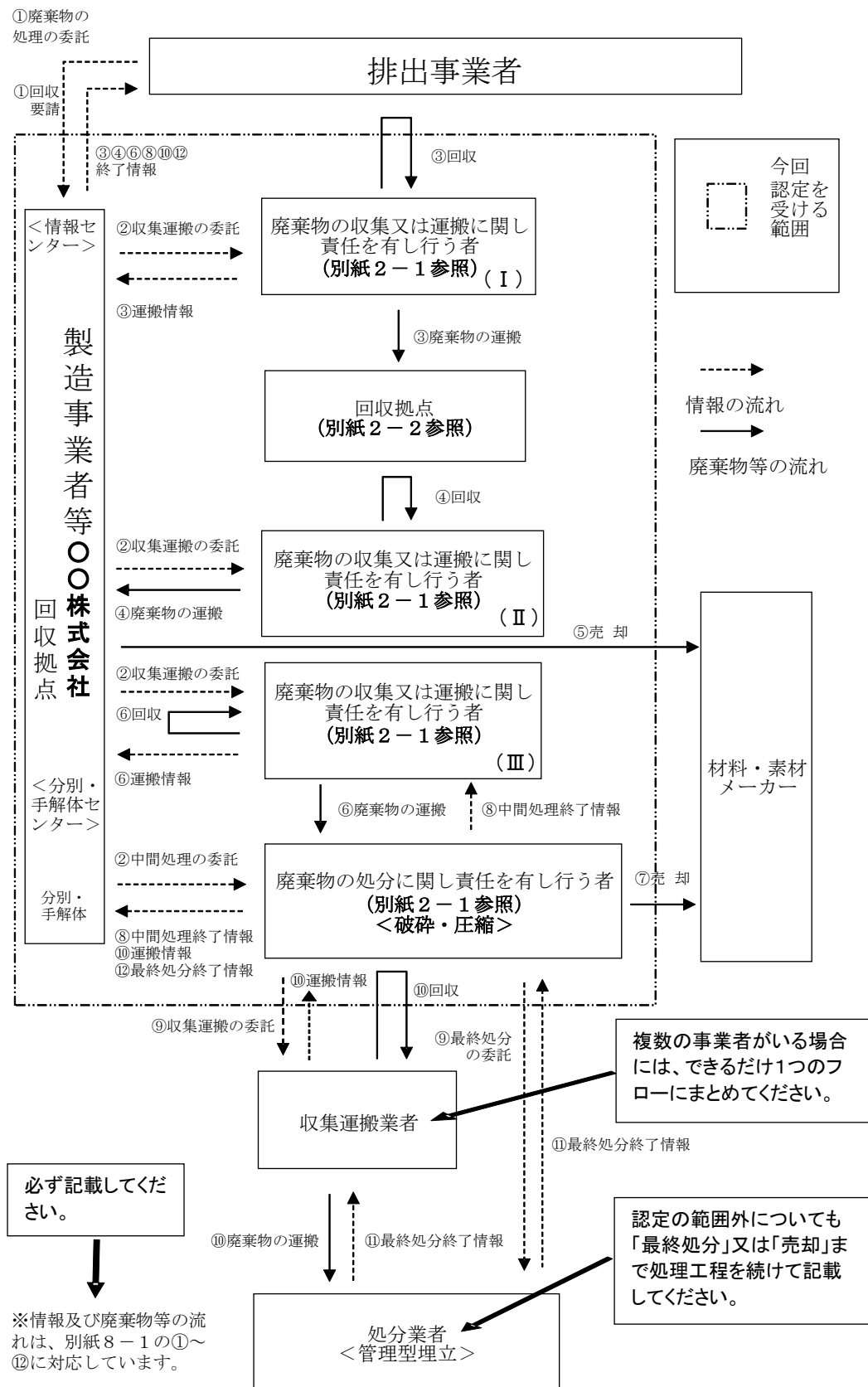
一連の処理の行程図
