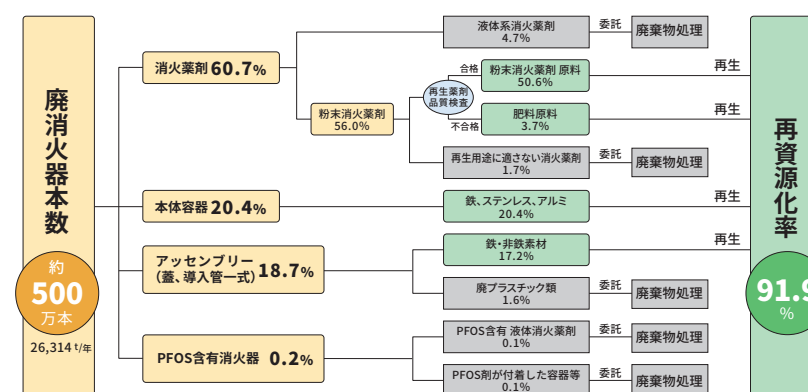
● 消火器リサイクルの MATERIAL FLOW (2022年度実績)
